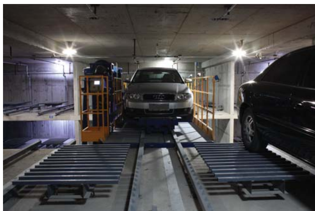
Рис. 5. Гребенчатая система хранения автомобиля
